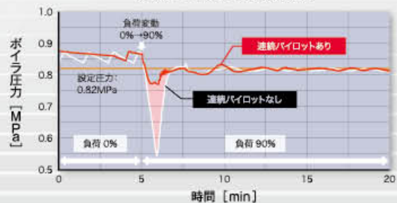
連続パイロット時負荷追従性
