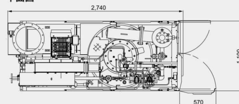
平面図
