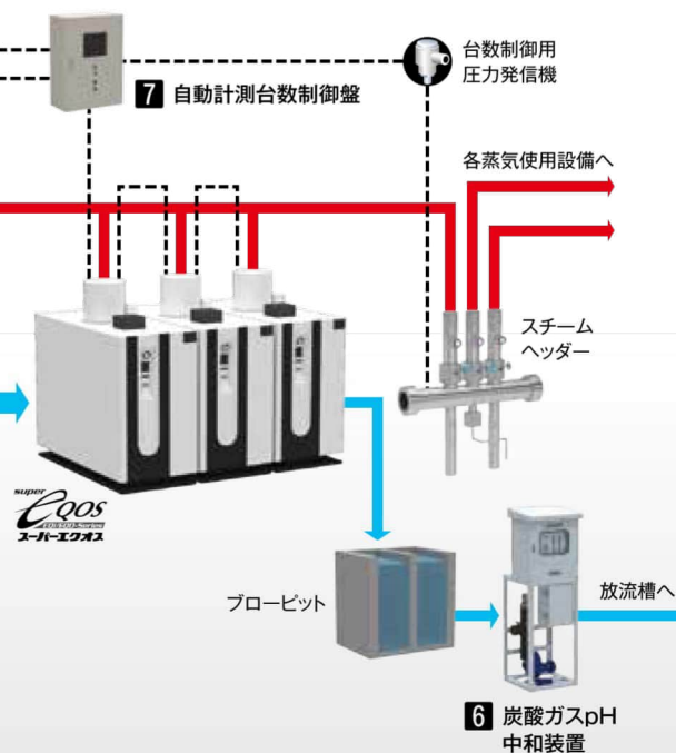
遠隔監視システム
