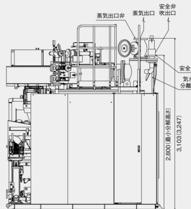
側面図
