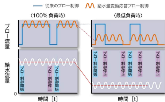
ブロー制御
