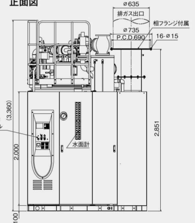
正面図
