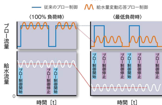
ブロー制御
