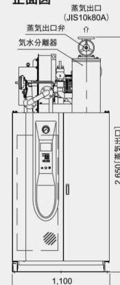
正面図
